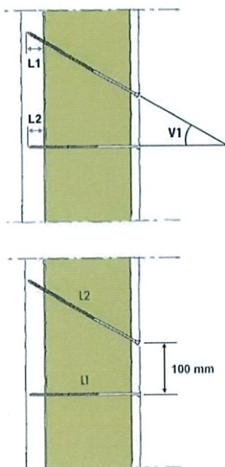
Fig. 3 Plassering av skrårskruene. Figur: Paroc AB
