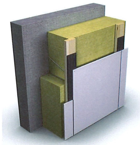
Fig. 2 Prinsipiell utførelse av PAROC ZEROfix montert på veggkonstruksjon av betong. Eksempel med utvendig platekledning. Figur: Paroc AB
