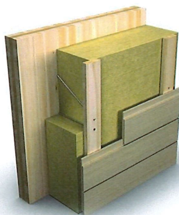
Fig. 1 Prinsipiell utførelse av PAROC ZEROfix montert på veggkonstruksjon av massivtre. Eksempel med utvendig trekledning. Figur: Paroc AB
