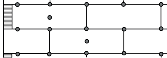
6 Dübel/m 2
