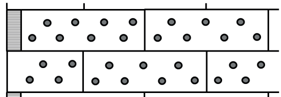
16 Dübel/m 2
