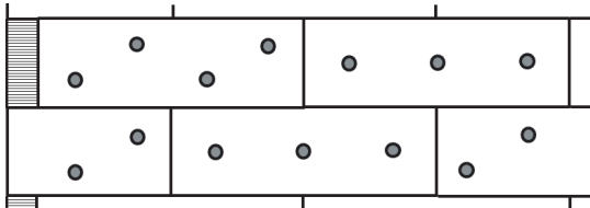
8 Dübel/m 2
