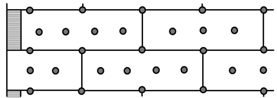
12 Dübel/m 2
